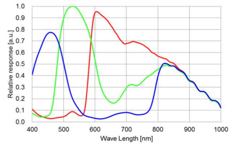
IMX307 分光感度
