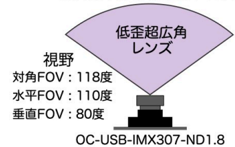
ND1.8 EFL : 1.8mm F : 2.4
