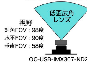
ND2.8 EFL : 2.8mm F : 4.0
