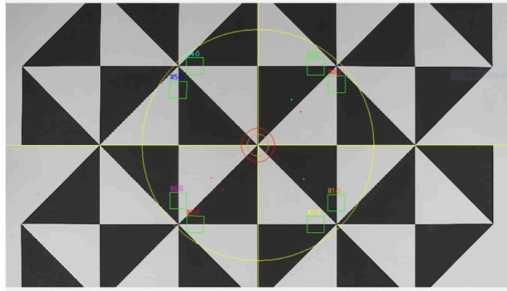
【OC-USB-IMX307-ND8.0 OctaTester評価 像高0.7F Sagital】
