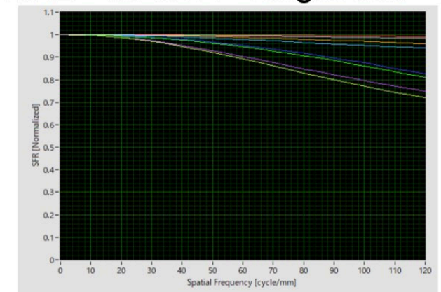
【OC-USB-IMX307-ND8.0 OctaTester評価 像高0.7F Tangential】
