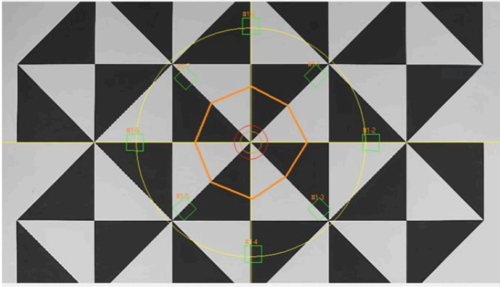
【OC-USB-IMX307-ND8.0 OctaTester評価 像高0.4F Tangential】
