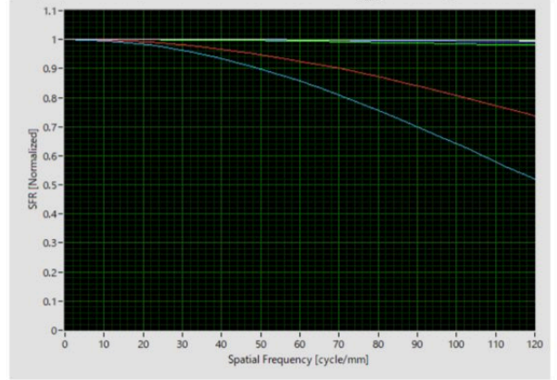
【OC-USB-IMX307-ND8.0 OctaTester評価 像高0.4F Tangential】
