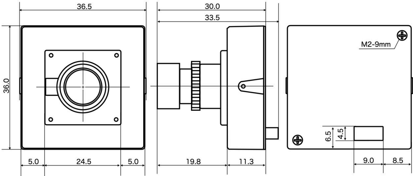
【三脚取付図】
