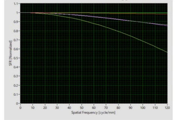
【OC-USB-IMX307-ND8.0 OctaTester評価 像高0.7F Sagital】
